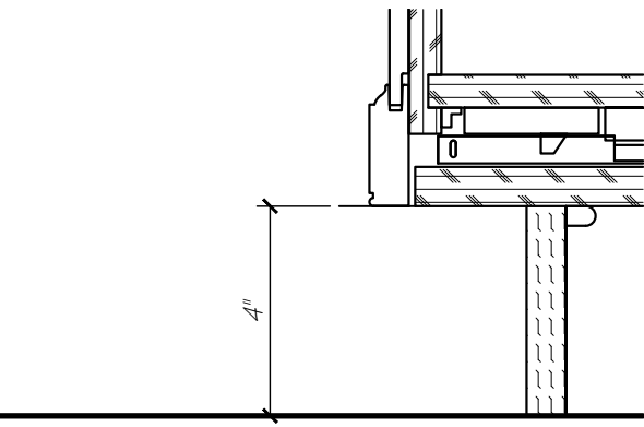
TOE DETAIL ✓ SCALE: 3" = 1'-0"
