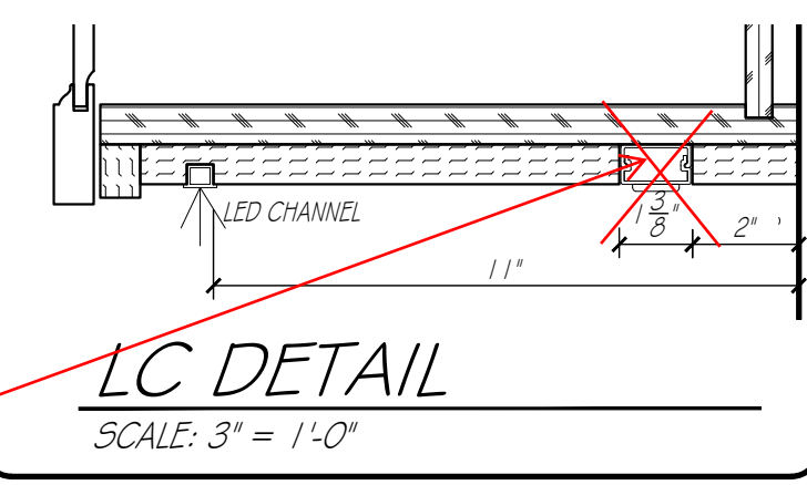
CROWN DETAIL SCALE: 3" = 1'-0"
