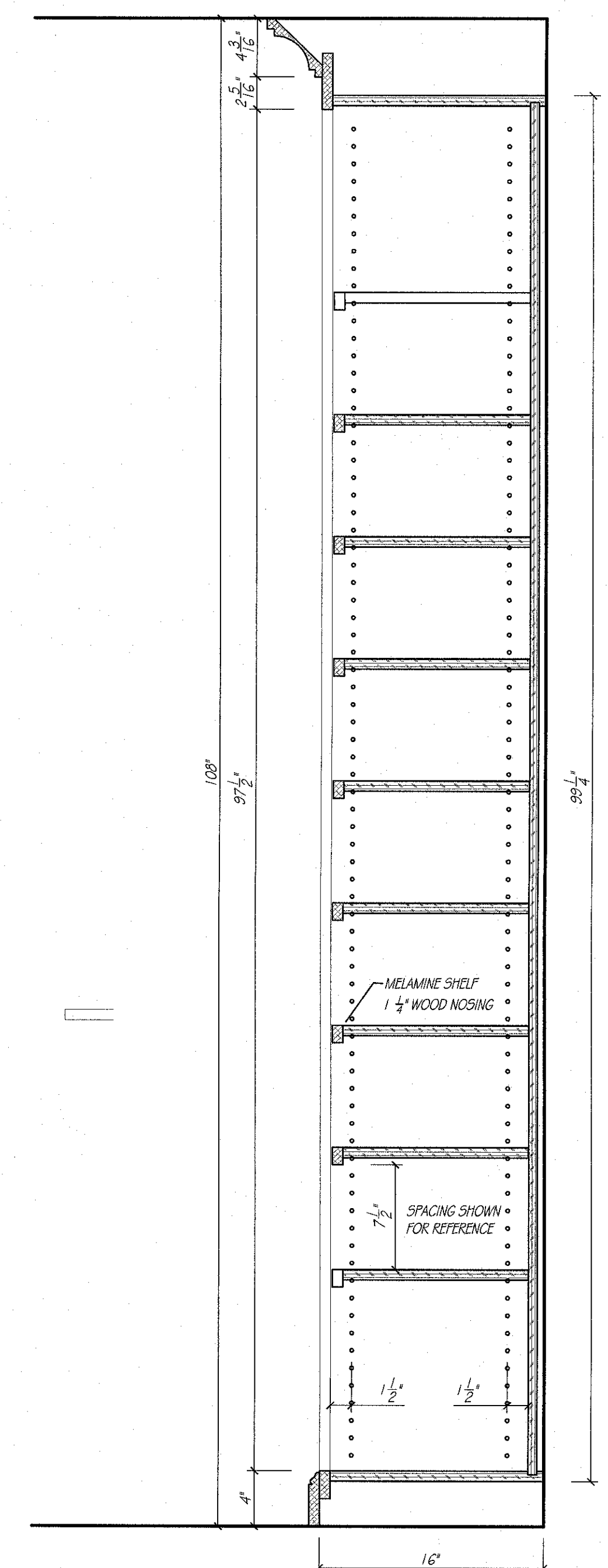
9 A11 CABINET DETAIL SCALE: 1 1/2" = 1'-0"
