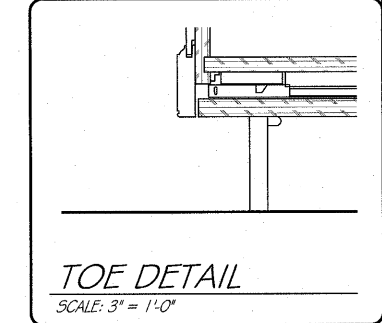
LC DETAIL SCALE: 3" = 1'-0"
