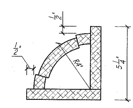
RADIUS CORNER DETAIL SCALE: 3" = 1'-0"
