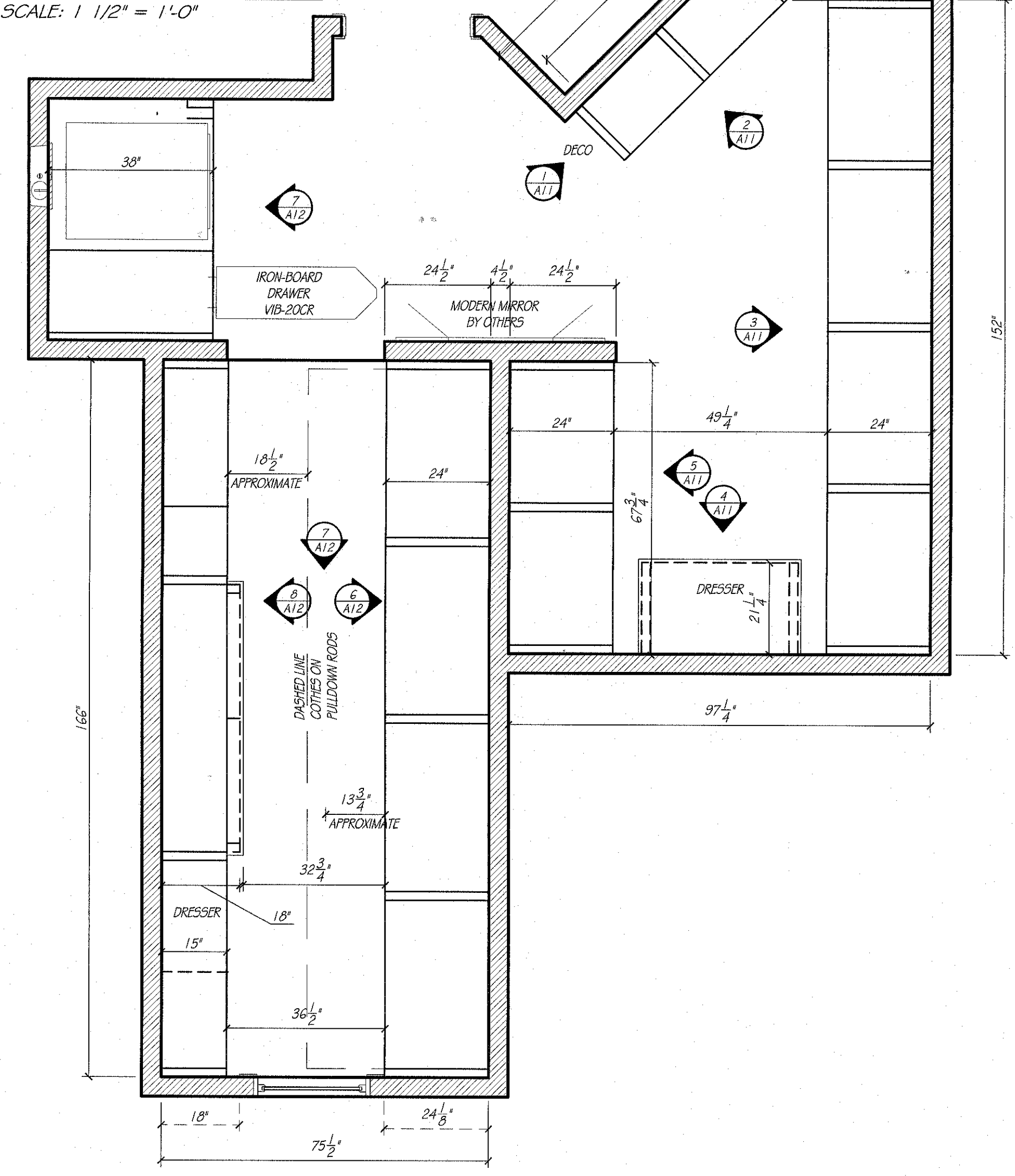
PRIMARY WARDROBE SCALE: 1/2" = 1' - 0"
