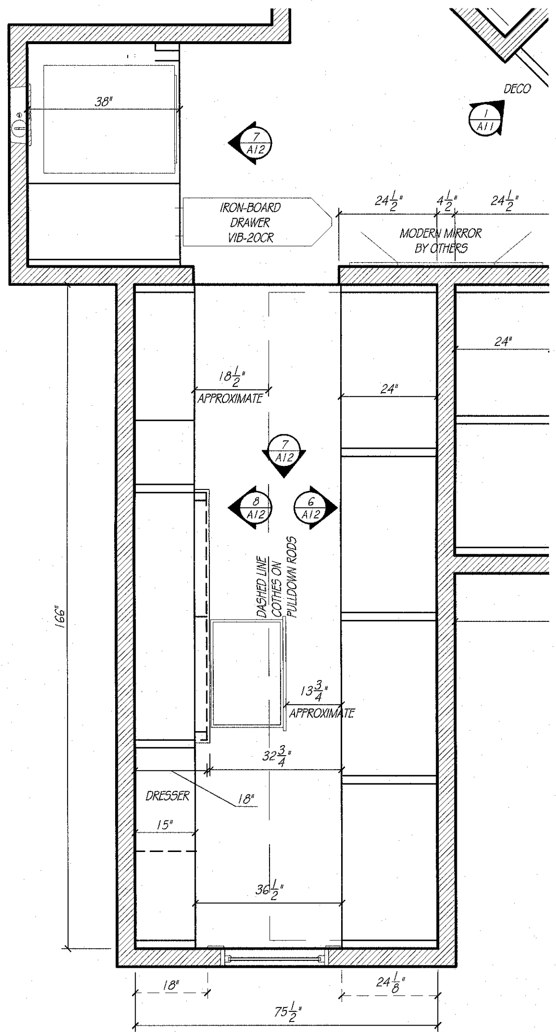
PRIMARY WARDROBE SCALE: 1/2" = 1'-0"
