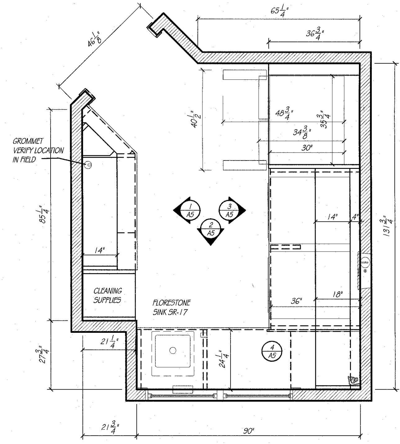
LAUNDRY SCALE: 1/2" = 1'-0"
