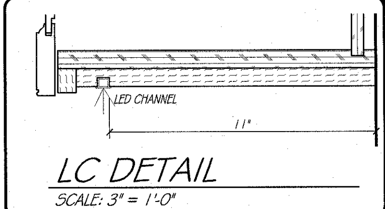
CROWN DETAIL SCALE: 3" = 1'-0"
