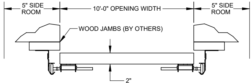
JAMB DETAIL
