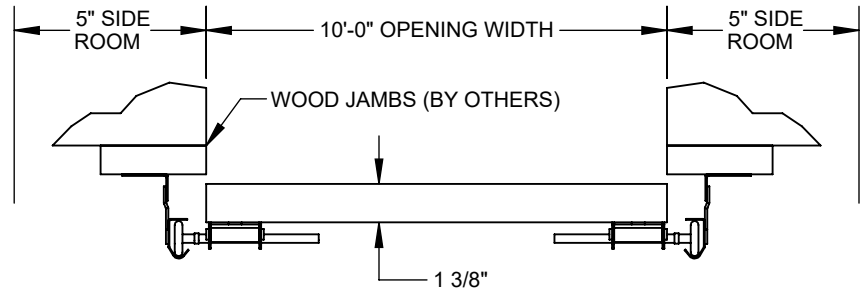
JAMB DETAIL
