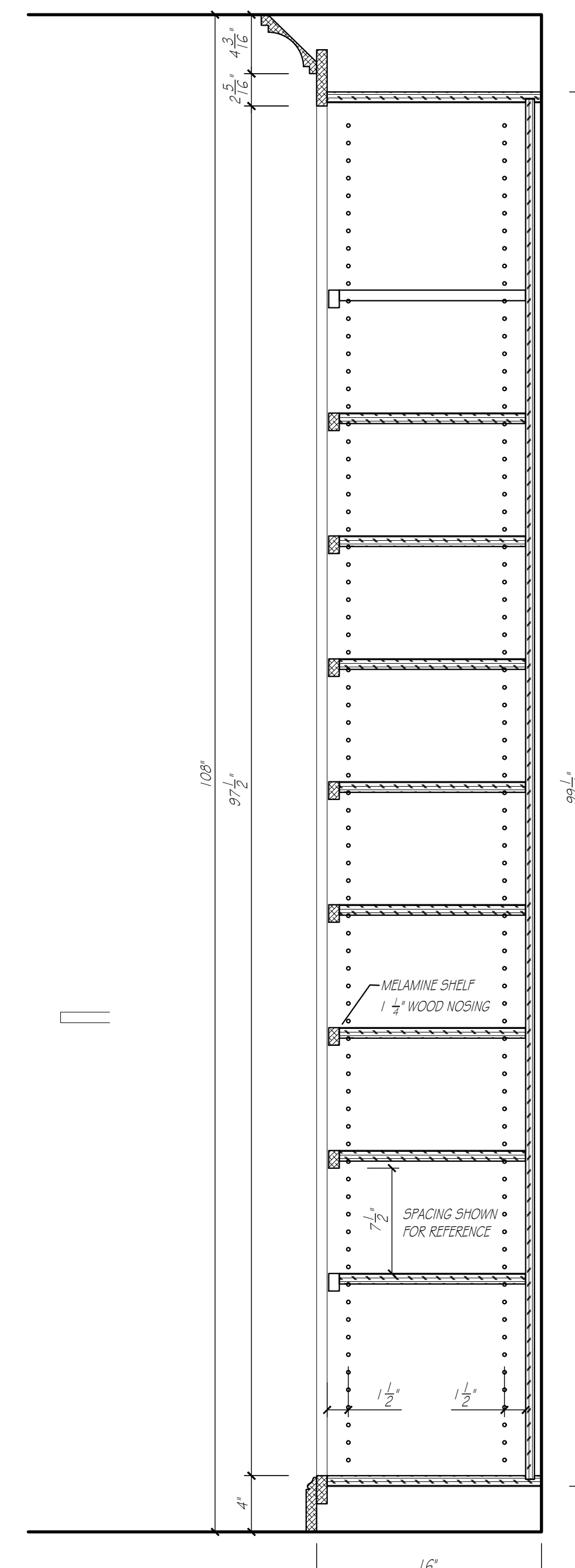
9 A11 CABINET DETAIL SCALE: 1 1/2" = 1'-0"
