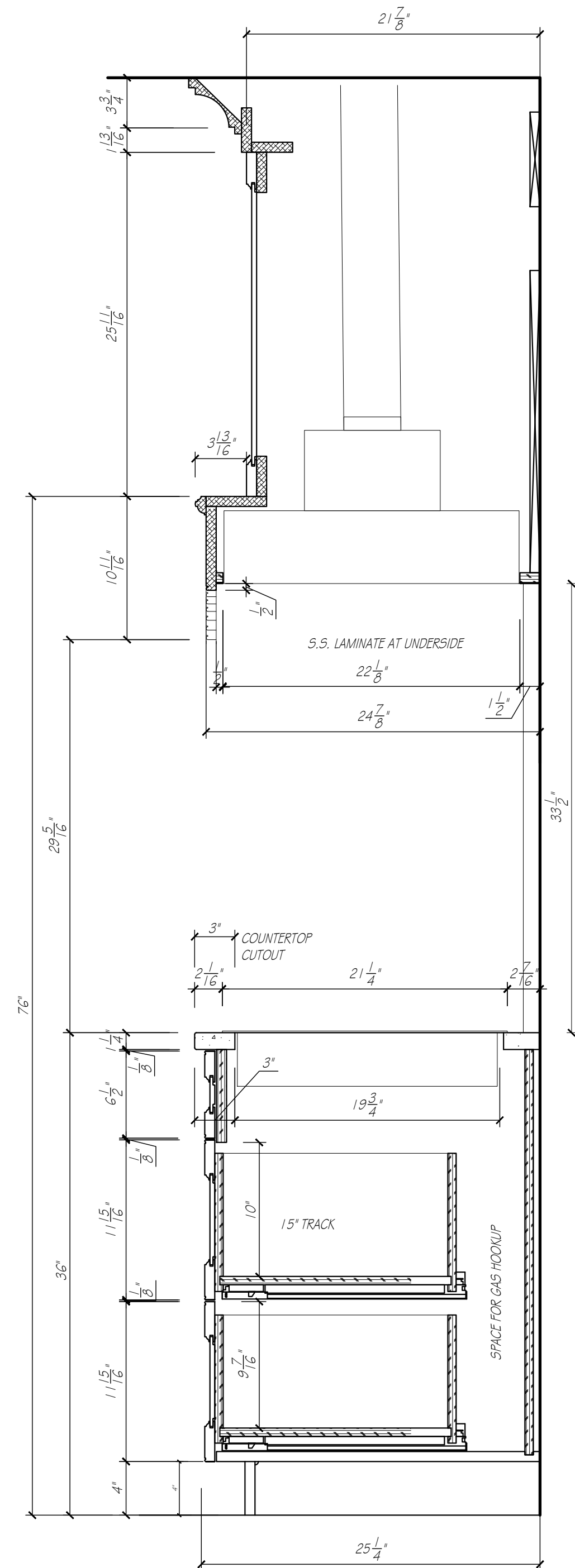
10 A3 CABINET DETAIL SCALE: 1 1/2" = 1'-0"
