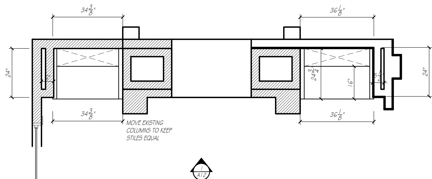
HEARTH ROOM SCALE: 1/2" = 1'-0"
