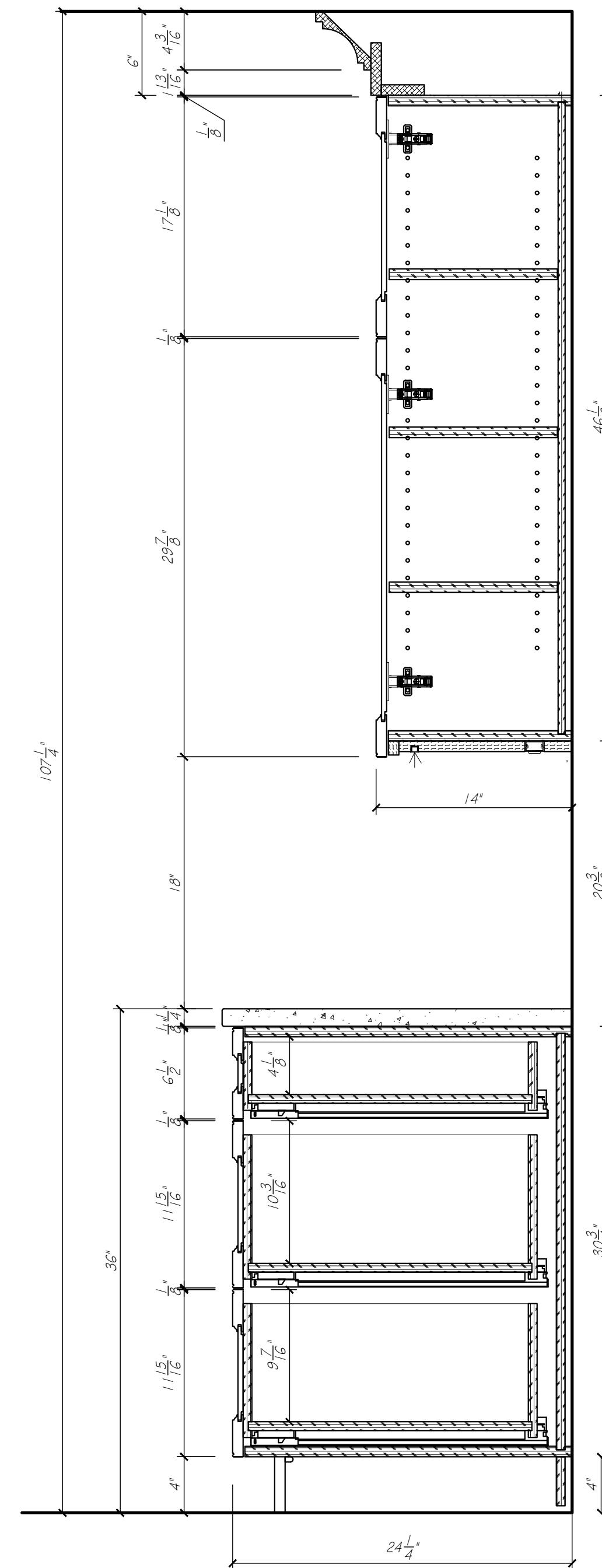
11 A3 CABINET DETAIL SCALE: 1 1/2" = 1'-0"
