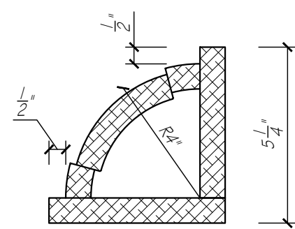
RADIUS CORNER DETAIL SCALE: 3" = 1'-0"
