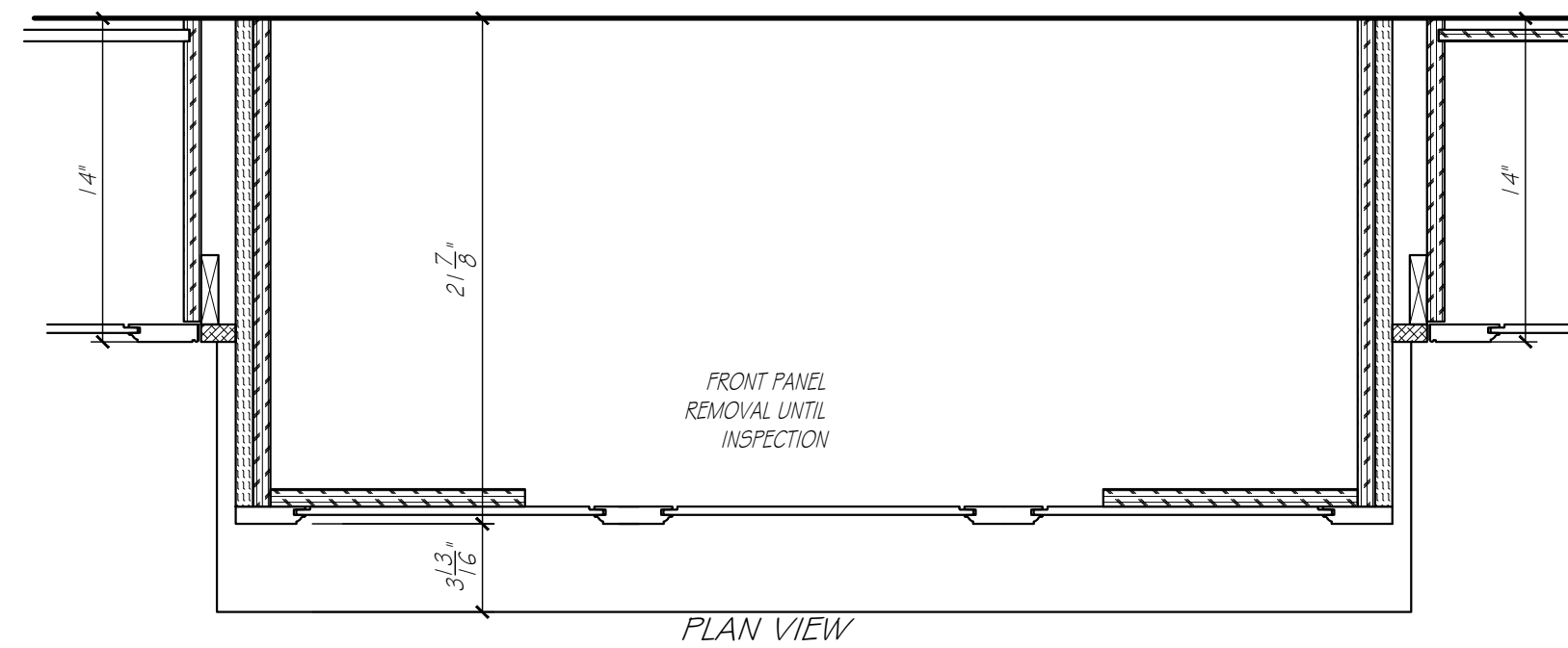
HOOD DETAIL SCALE: 1 1/2" = 1'-0"
