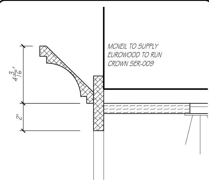
CROWN DETA.
