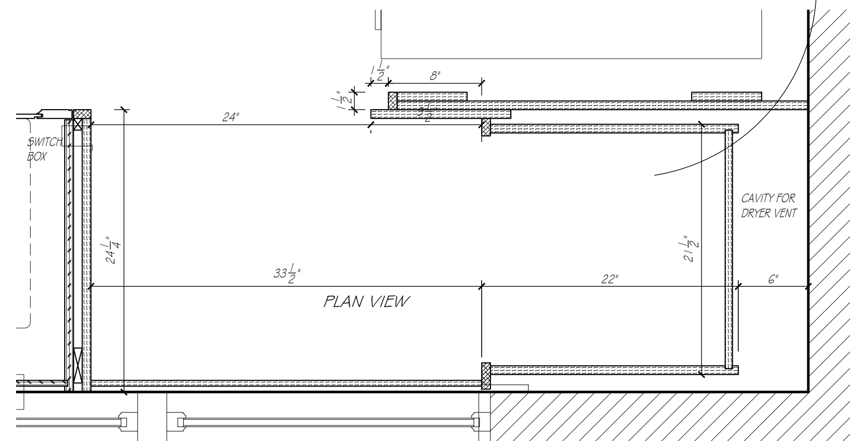
6 A5 CABINET DETAIL SCALE: 1 1/2" = 1'-0"
