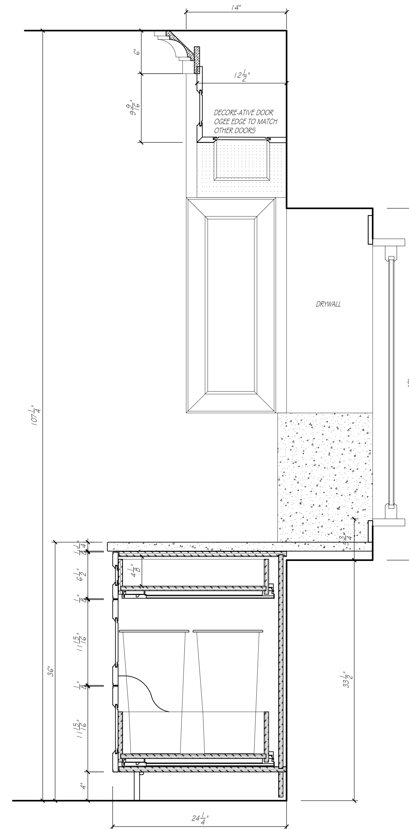
12 A3 CABINET DETAIL SCALE: 1 1/2" = 1'-0"
