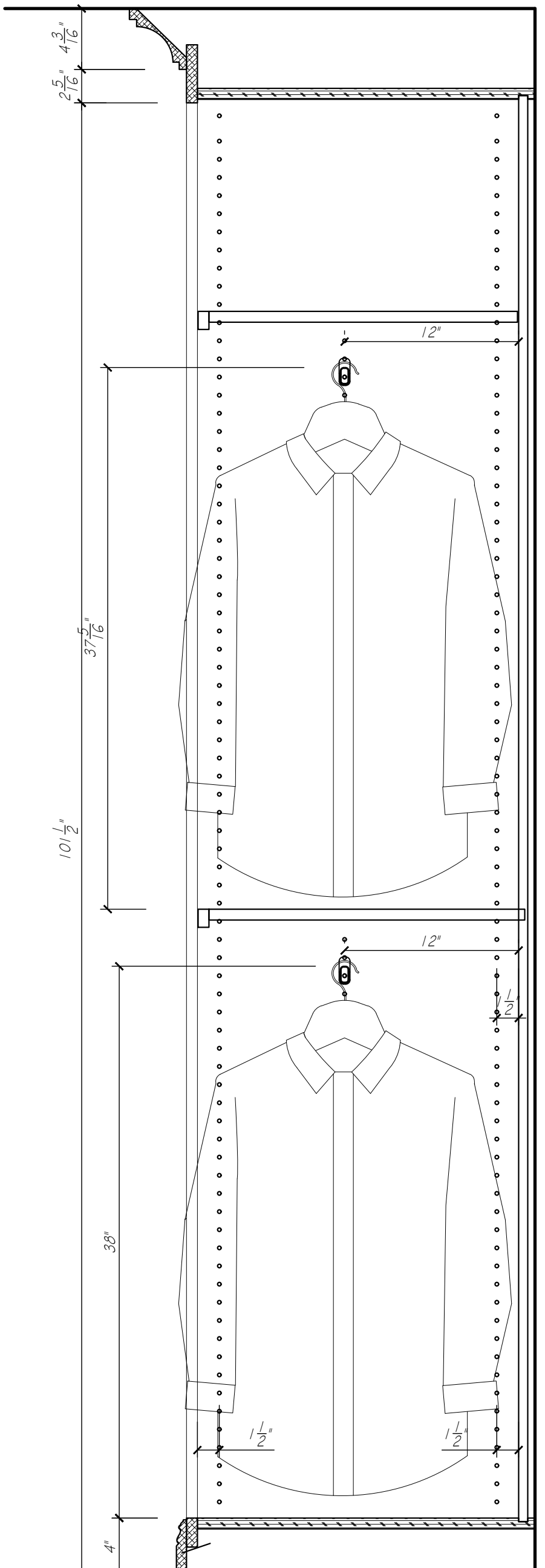
SCALE: 1 1/2" = 1'-0"
