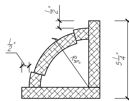
RADIUS CORNER DETAIL SCALE: 3" = 1'-0"
