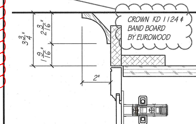
CROWN DETAIL SCALE: 3" = 1' - 0"
