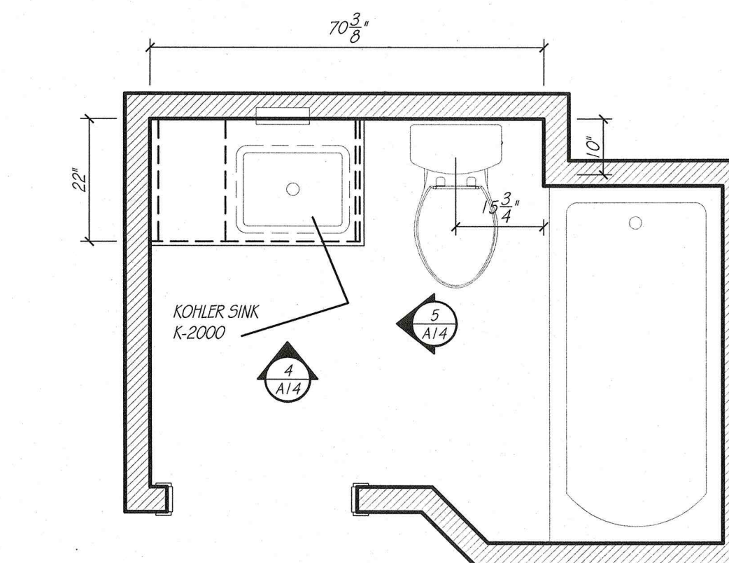
BATH 3 SCALE: 1/2" = 1' - 0"
