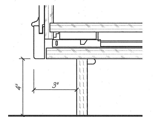
TOE DETAIL ✓ SCALE: 3" = 1'-0"
