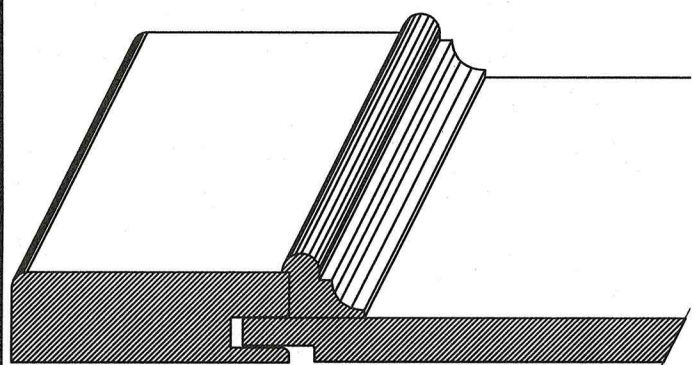
TOE DETAIL SCALE: 3\"/>
