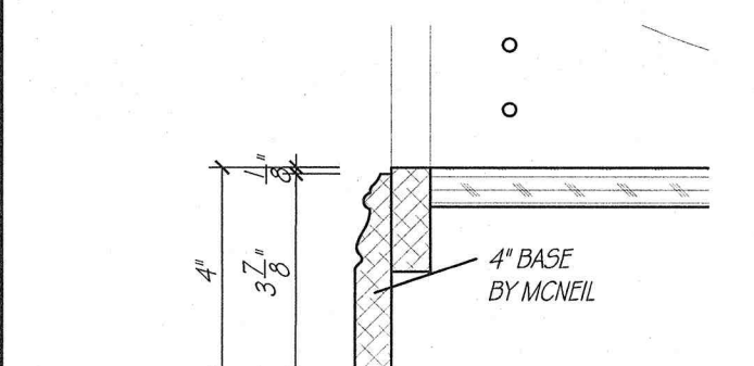
TOE DETAIL SCALE: 3\"/>
