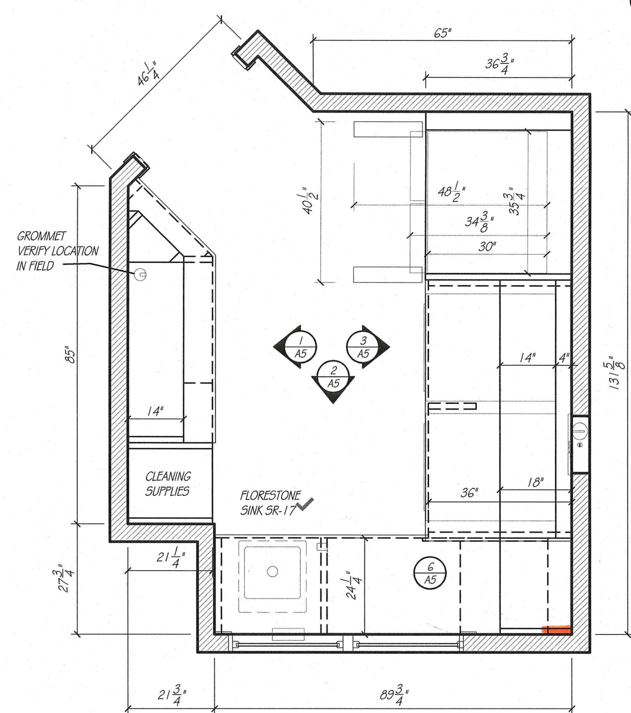
LAUNDRY SCALE: 1/2" = 1'-0"
