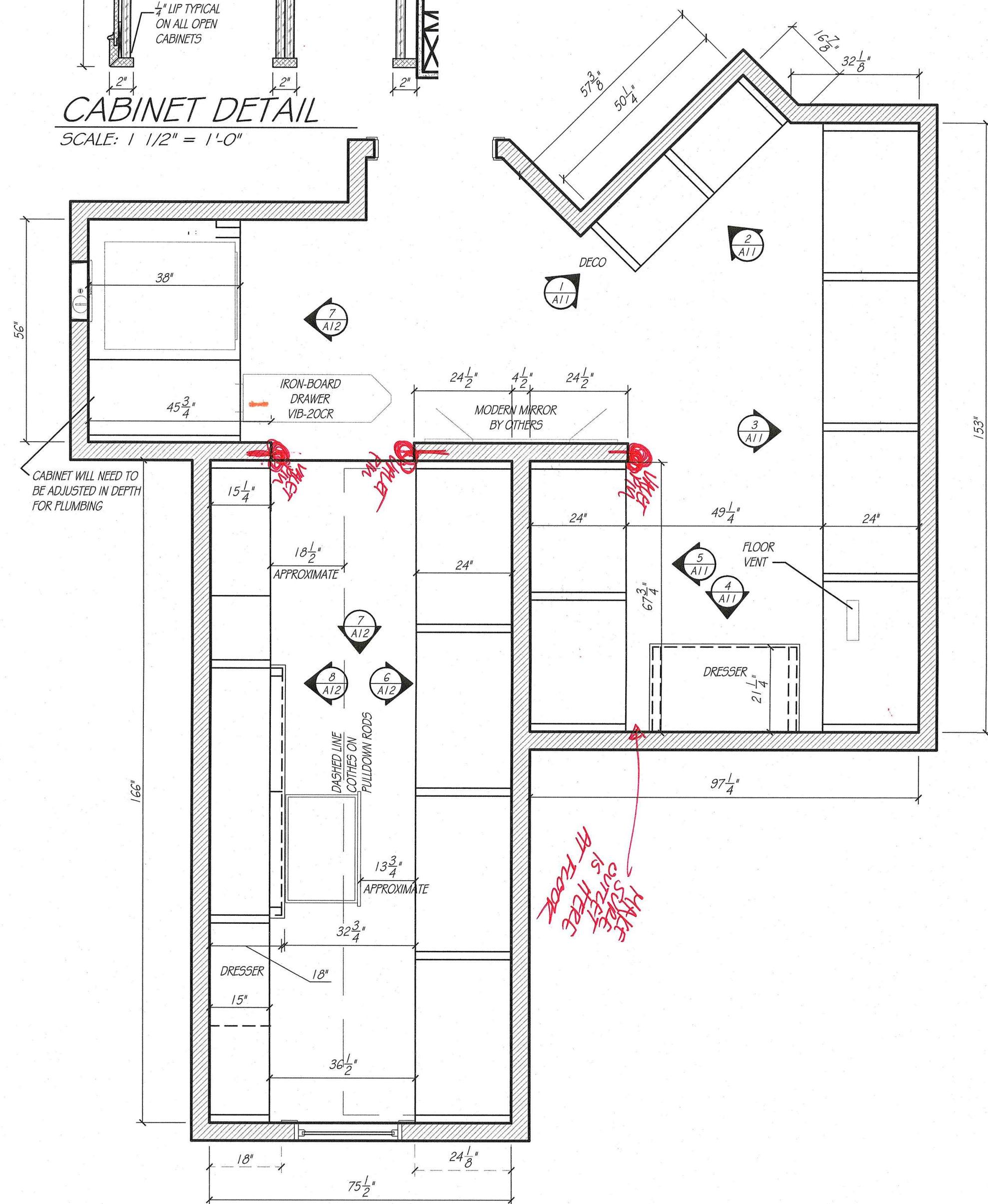
PRIMARY WARDROBE SCALE: 1/2" = 1'-0"
