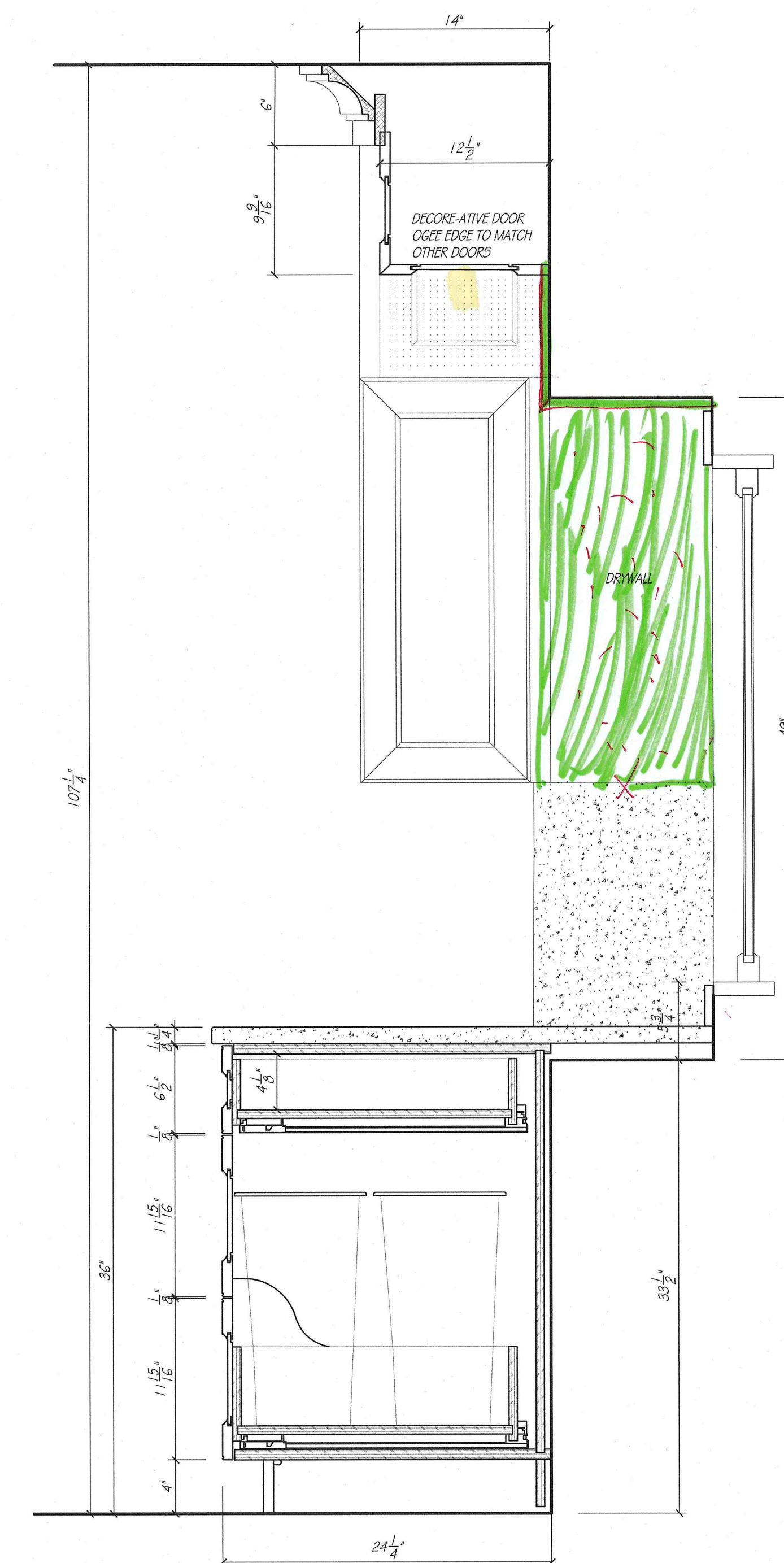
12 A3 CABINET DETAIL SCALE: 1 1/2" = 1'-0"
