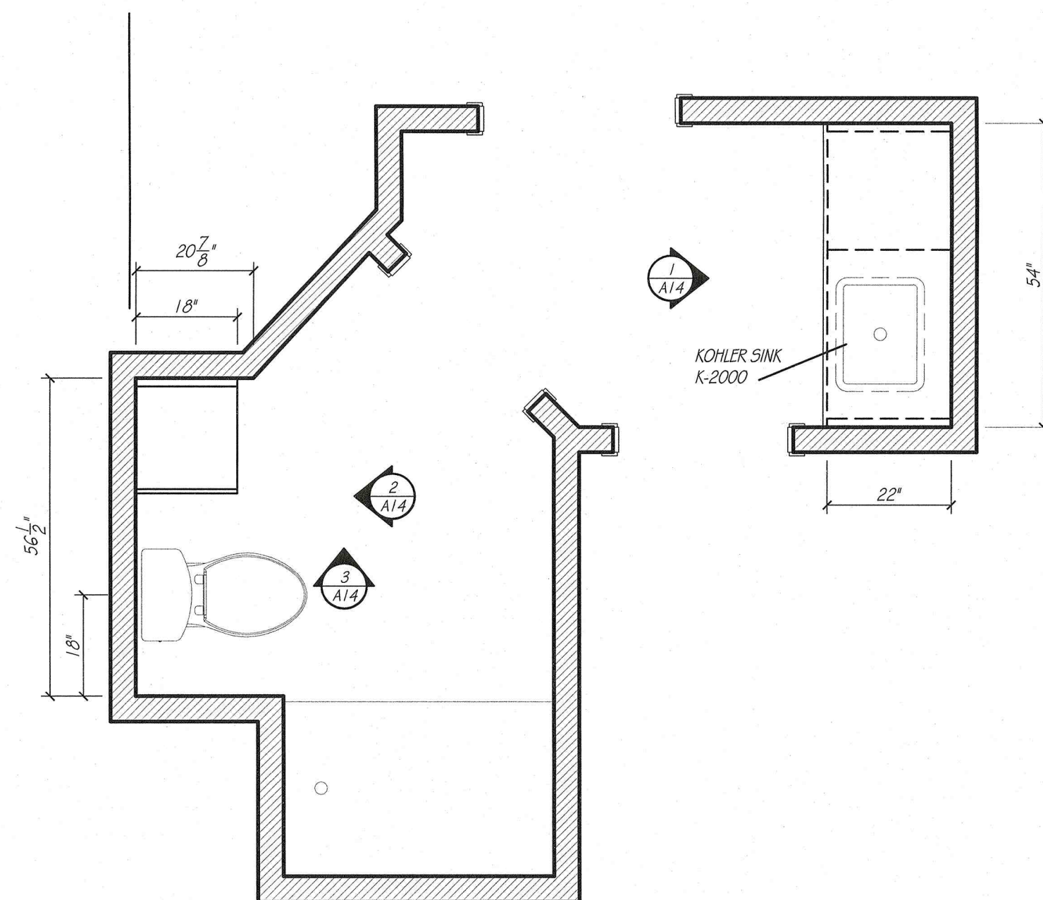
BATH 2 SCALE: 1/2" = 1' - 0"
