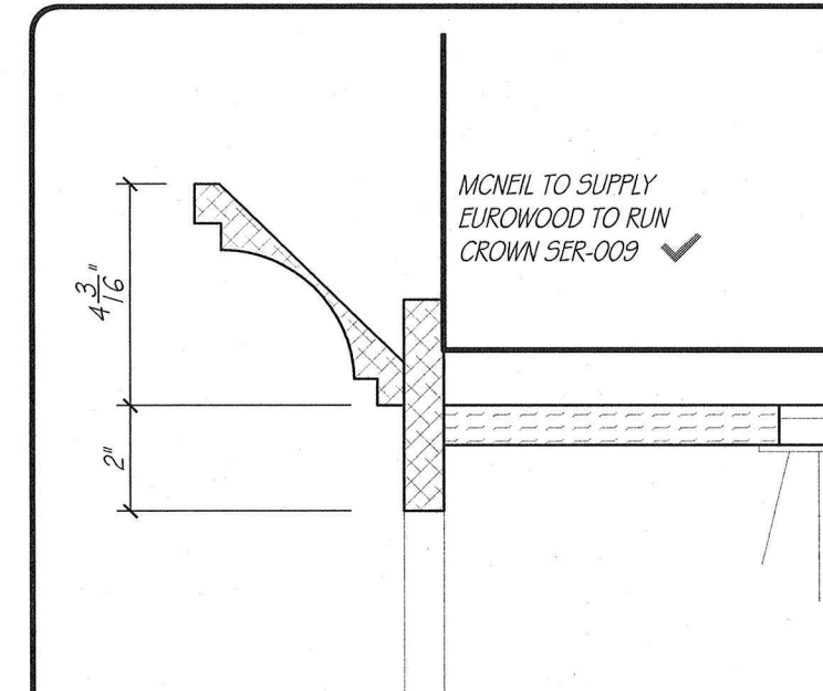
CROWN DETAIL SCALE: 3" = 1'-0"
