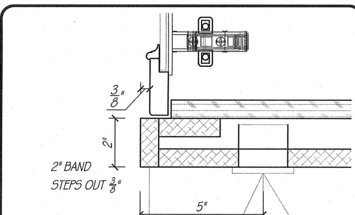
LC DETAIL SCALE: 3\"/>
