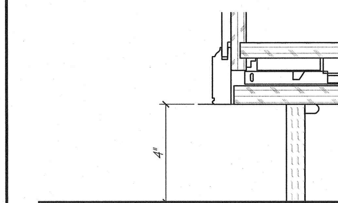
TOE DETAIL ✓ SCALE: 3" = 1' - 0"
